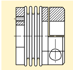
Tipo AKD/CK Tipo com cubo de fixação e flange
